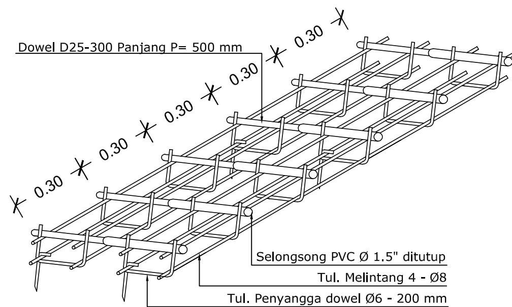
ISOMETRI PEMASANGAN DOWEL SKALA 1 : 10
