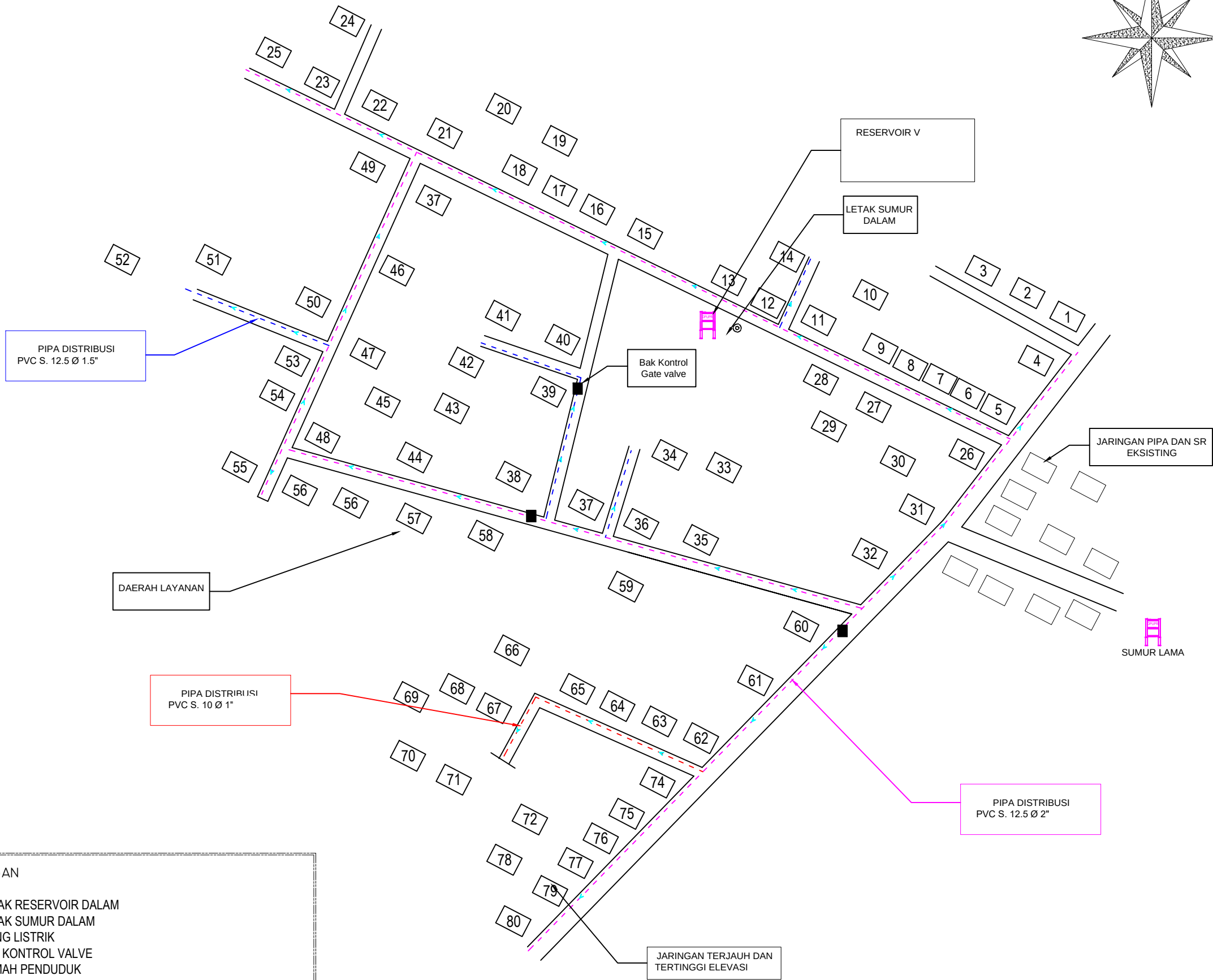
SITEPLAN PEMBANGUNAN SUMUR DALAM TERLINDUNG DESA KALIJIRAK KECAMATAN TASIKMADU
