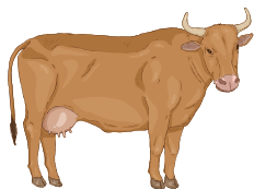
SAPI
