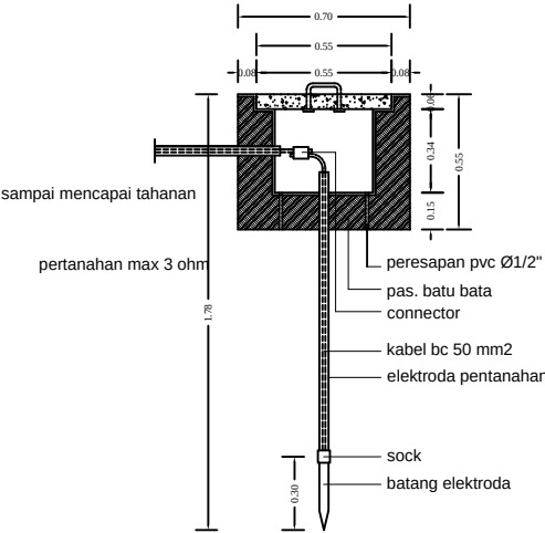
DETAIL BAK KONTROL SKALA 1: 25
