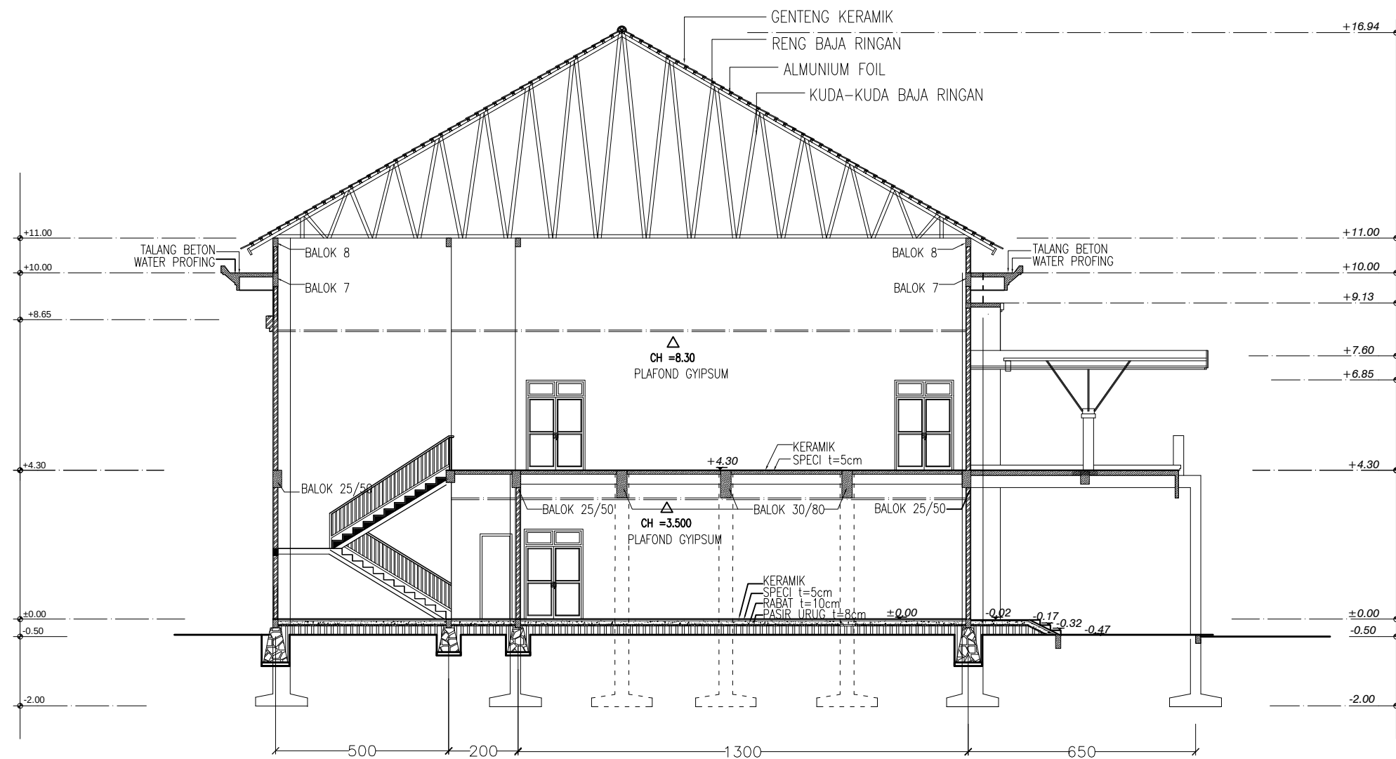
POTONGAN B-B skala 1 : 150
