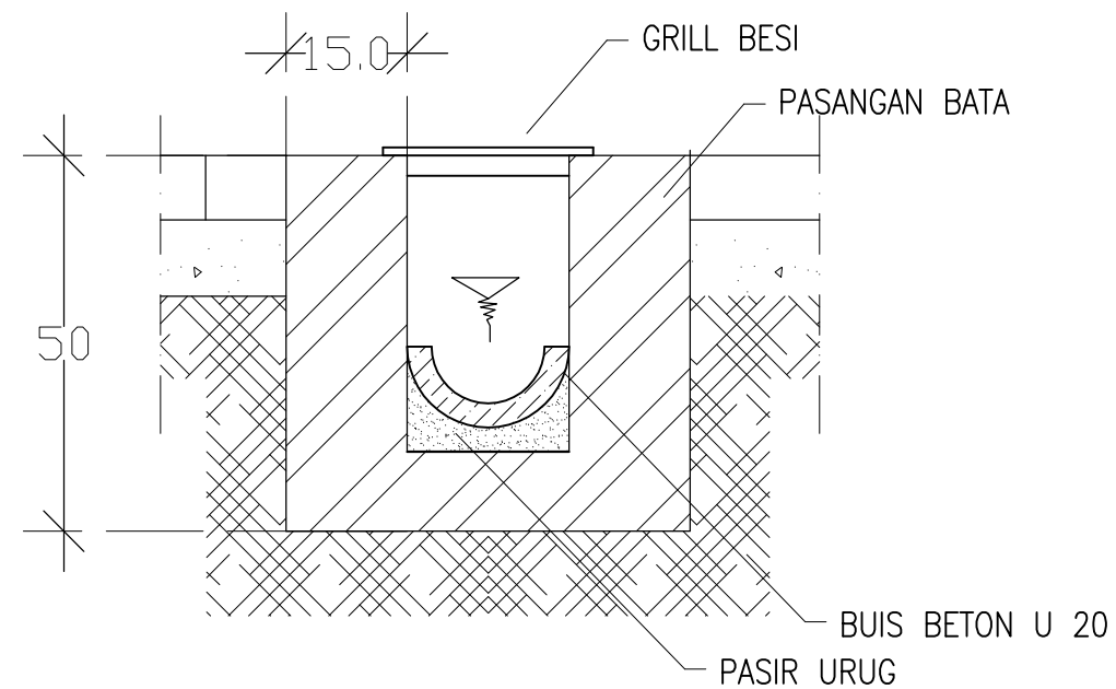
DETAIL SALURAN skala 1 : 10
