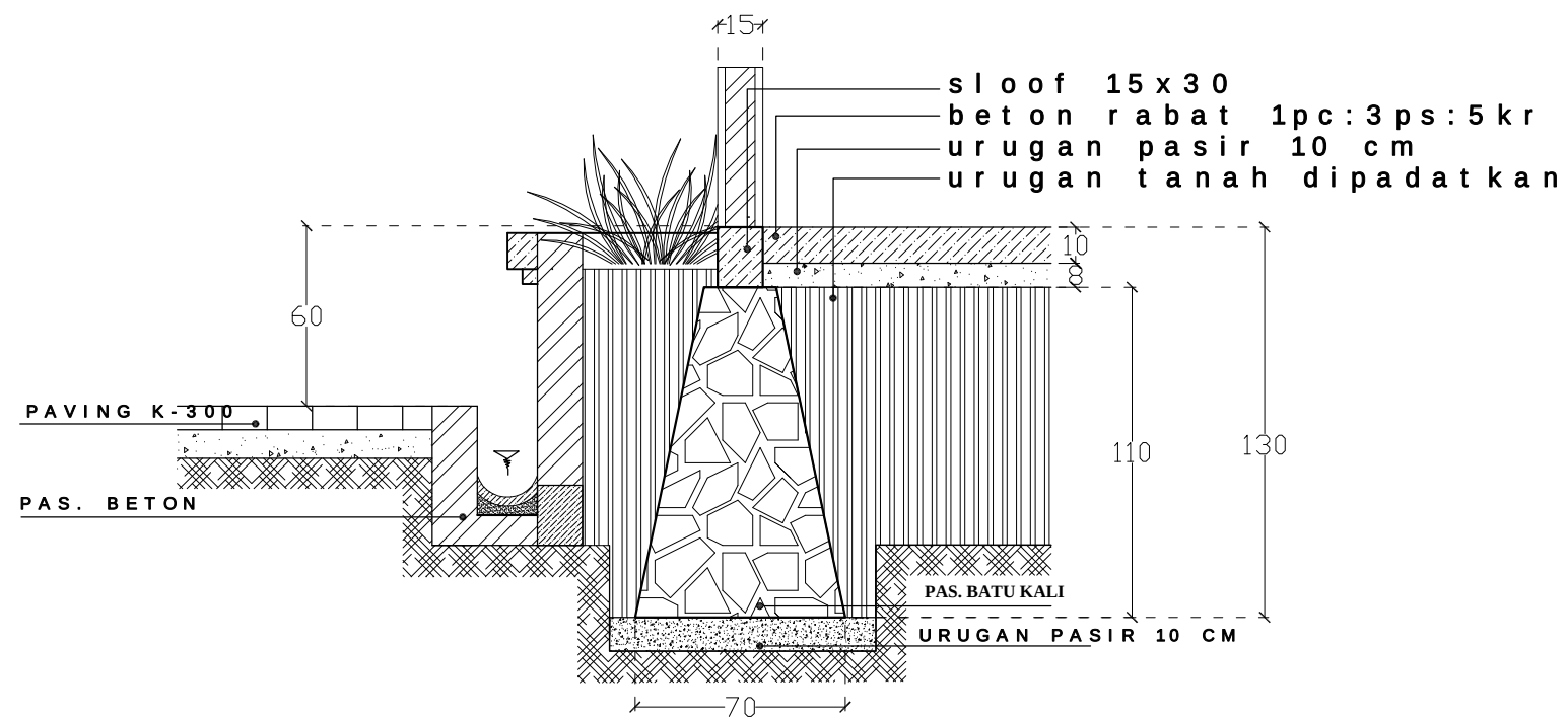
DETAIL PONDASI TEPI skala 1 : 25
