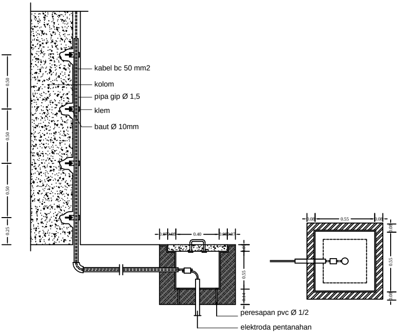
ELECTRODA PENYALUR PETIR (PP) SKALA 1: 25
