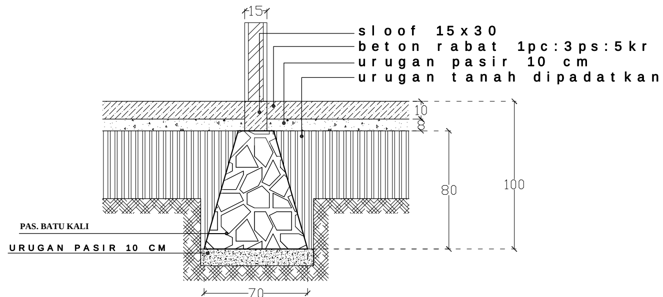
DETAIL PONDASI DALAM skala 1 : 25
