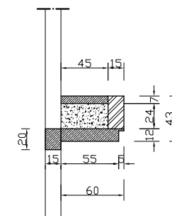
penampang 01 skala 1 : 50
