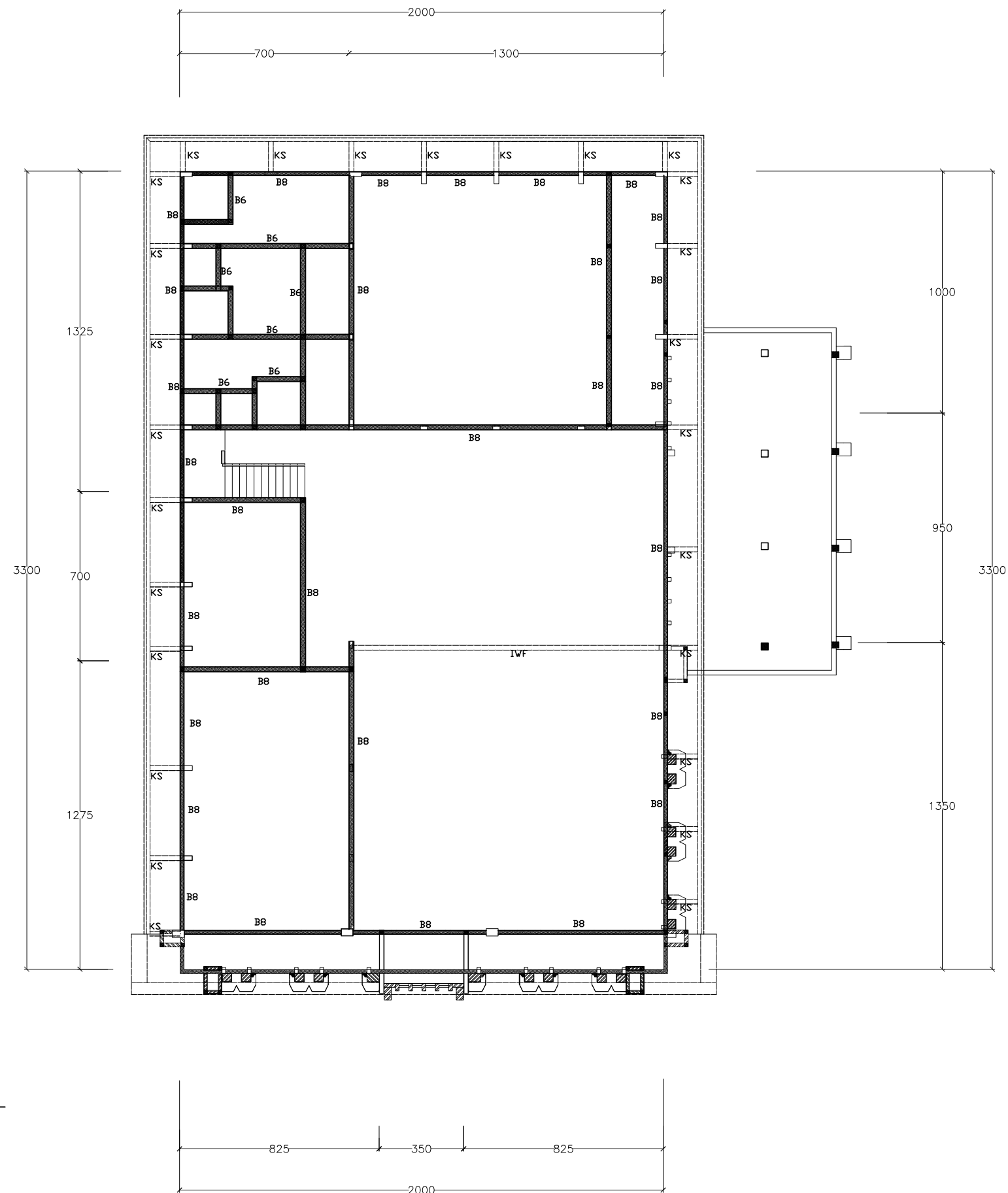
DENAH BALOK LANTAI 2 skala 1 : 200
