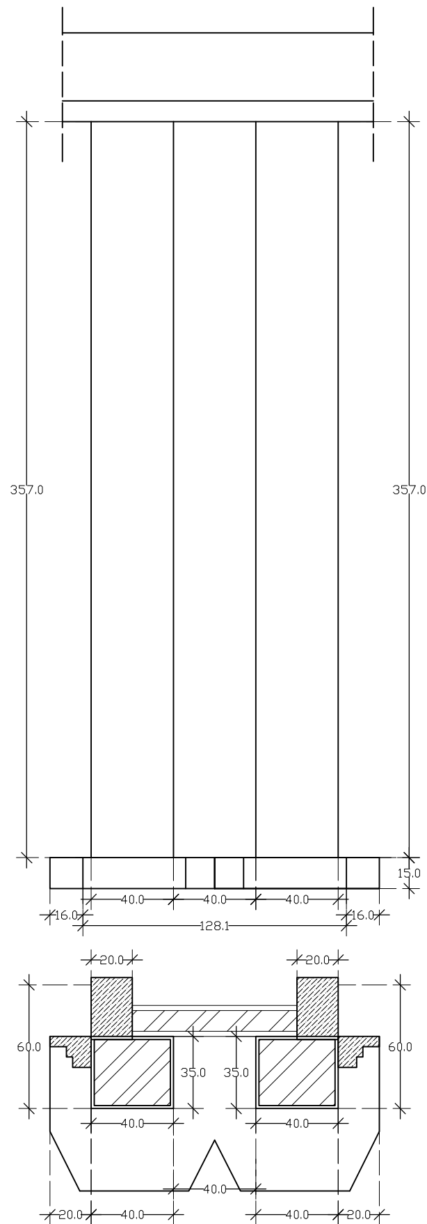
Penebalan Kolom lantai 2
