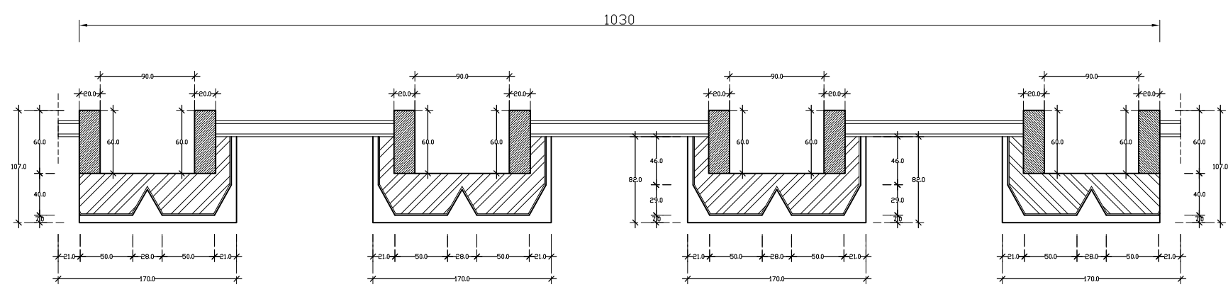
penampang B skala 1 : 50
