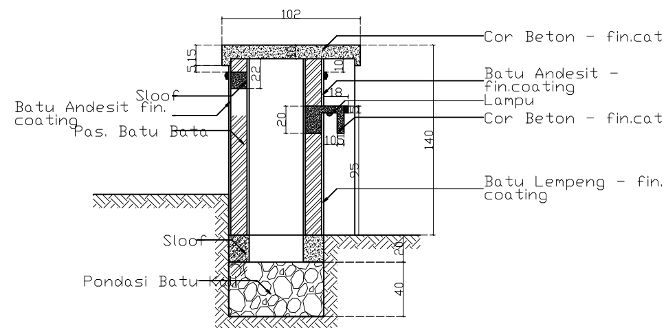
Potongan B-B skala 1 : 50
