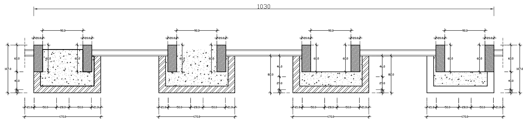
penampang C skala 1 : 50
