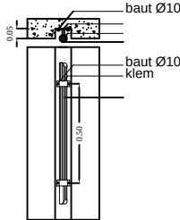
DETAIL KLEM DAN PEMASANGAN PIPA GIP SKALA 1: 25
