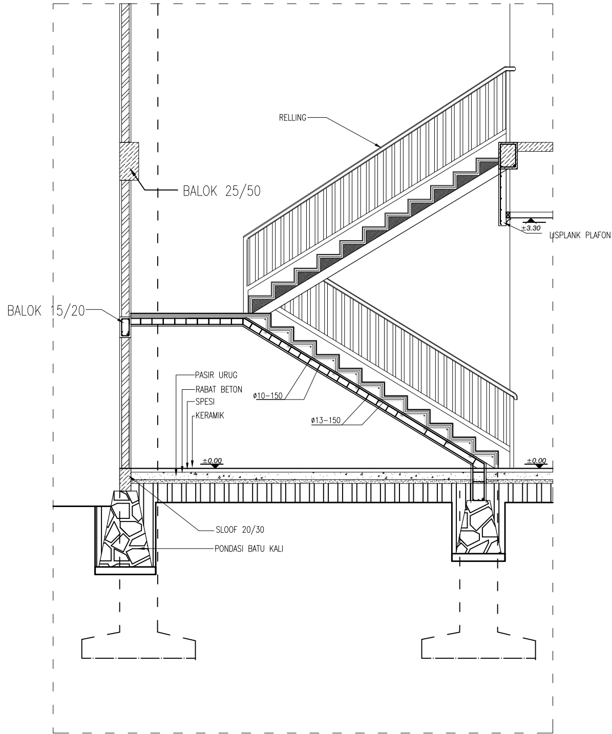
DETAIL TANGGA skala 1 : 50
