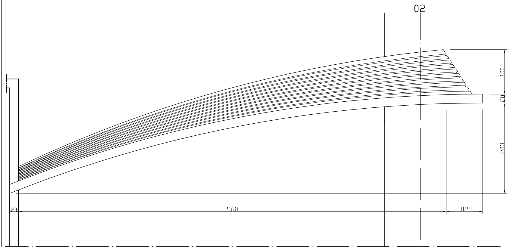
TAMPAK DEPAN VASADE 3 skala 1 : 50
