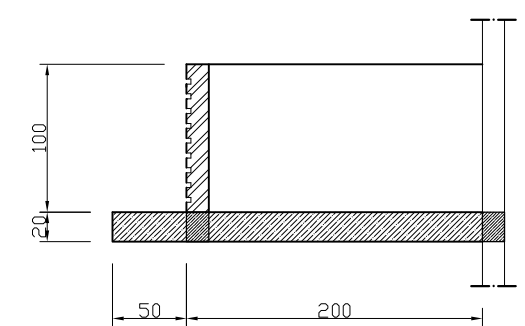
penampang 02 skala 1 : 50
