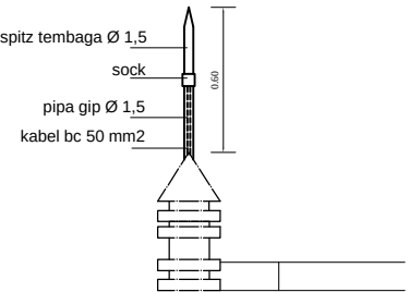
DETAIL PENEMPATAN SPITZ SKALA 1: 25
