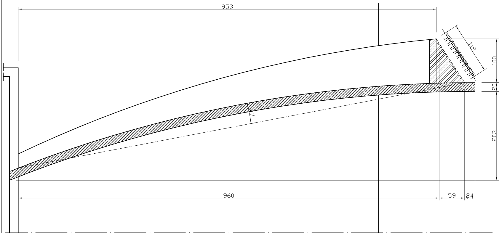
penampang 01 skala 1 : 50
