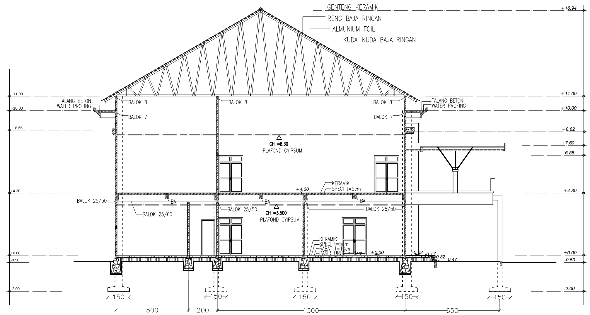
POTONGAN A-A skala 1 : 150
