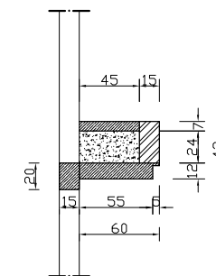
penampang 01 skala 1 : 50
