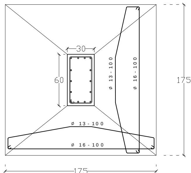
DETAIL PENUL. K1&P1 skala 1 : 20
