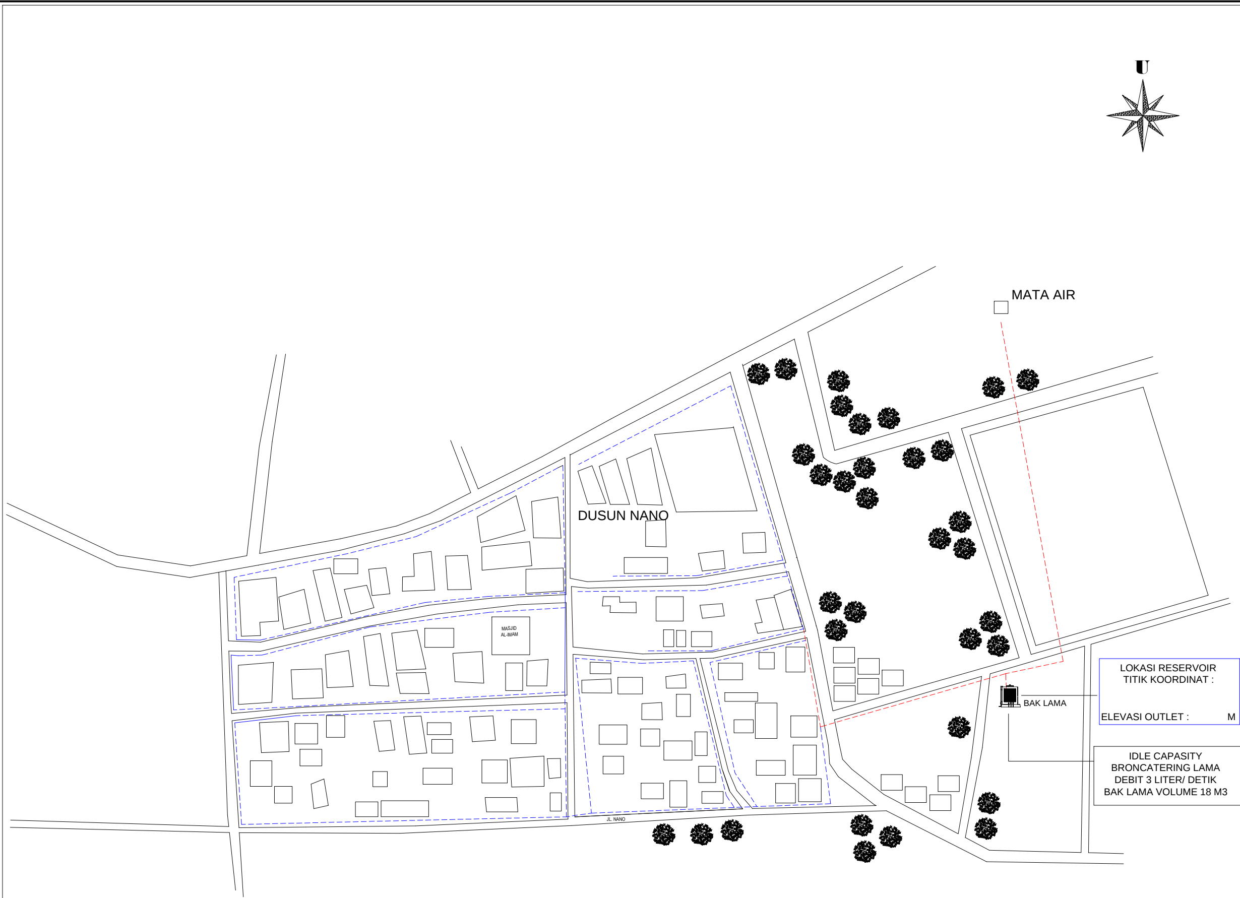
PETA LOKASI PENGEMBANGAN JARINGAN DISTRIBUSI DAN SAMBUNGAN RUMAH (SR) DUSUN NANO DESA TAWANGMANGU KECAMATAN TAWANGMANGU
